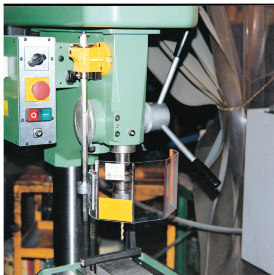
Dispositif de sécurité pour perceuses
