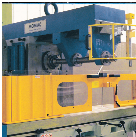
Dispositif de sécurité pour fraiseuses
